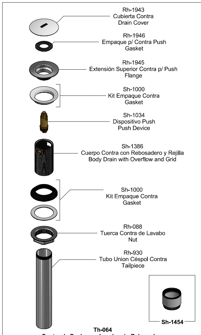
Th-064 Contra de Push para Lavabo sin Rebosadero Push Drain Lavatory without Overflow
