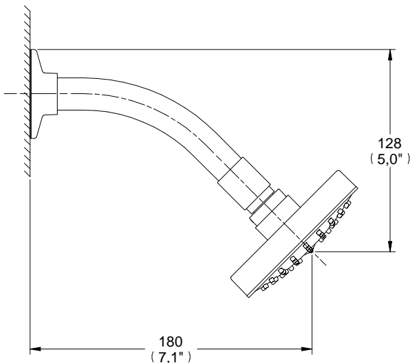
Medidas Referenciales/Estimated Dimensions, Acot.mm.(pulg)/Dim.mm.(in)
